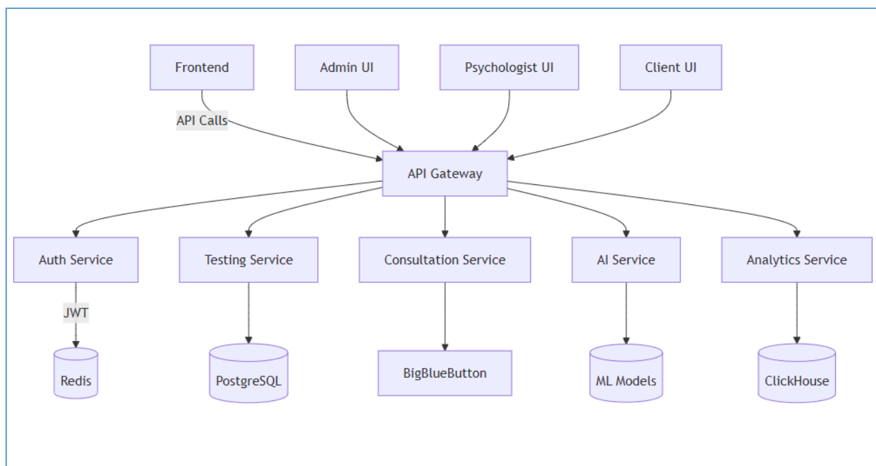
Рисунок 15 – Компонентная диаграмма
