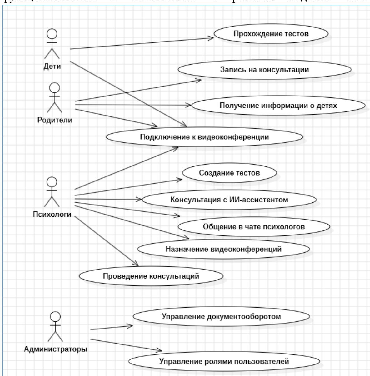
Рисунок 13 – Use-Case диаграмма
