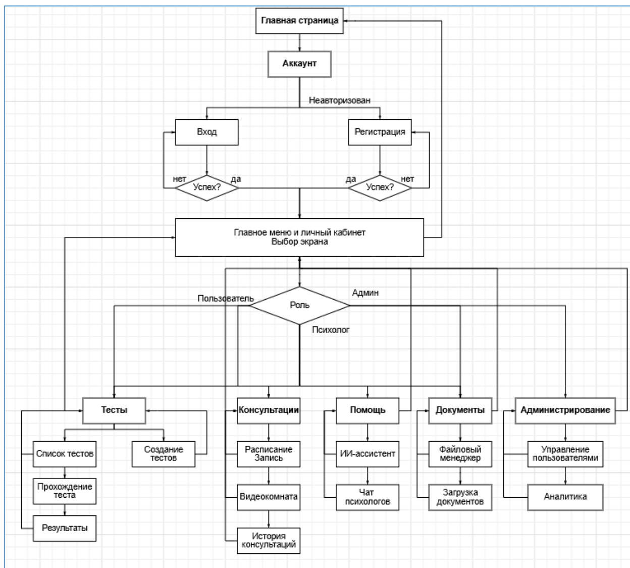
Рисунок 29 – Карта экранов
